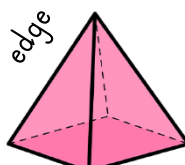
pyramid
