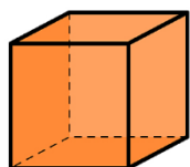
vertex
